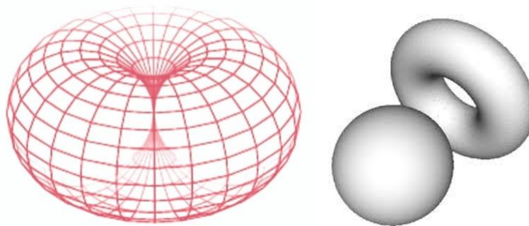
Slika 4: Na levi vidimo 3D rotacijsko polje pred transformacijo v kroglo, na desni pa sta obliki obeh skrajnih točk transformacije, ki ne bi mogli nastati brez časovne dimenzije.
